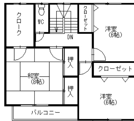
2階平面図
